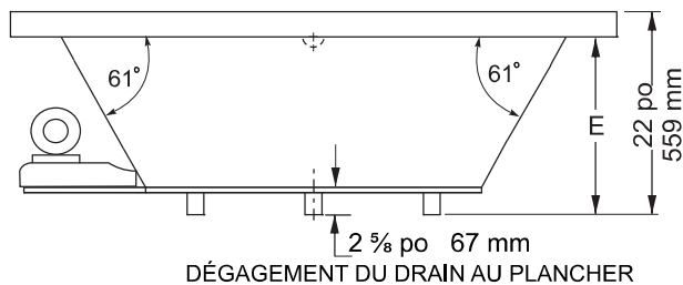
DÉGAGEMENT DU DRAIN AU PLANCHER
